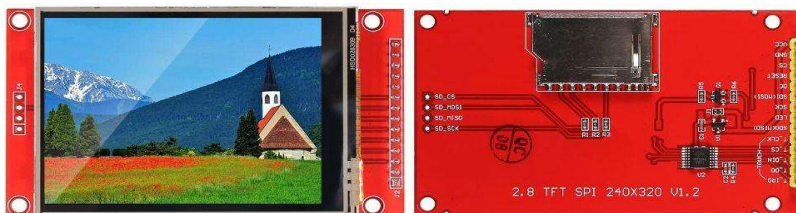
Display Lcd color TFT 2.2 240x320 Spi con SD
