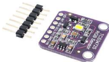
Sensor De Color Rgb Con Filtro TCS- 34725
