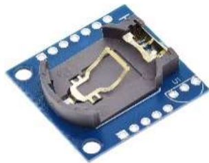
Modulo DS1307
