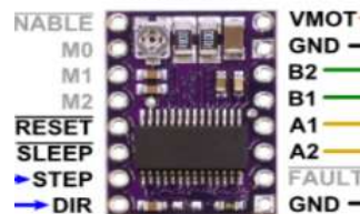
DRV8825
