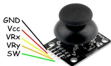
JOYSTICK ARDUINO
