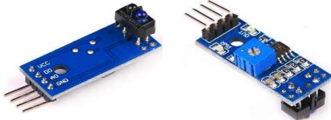
Seguidor de Lineas TCRT-5000
