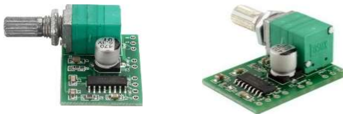
PAM 8403 Audio con Potenciometro 3+3w - 5v
