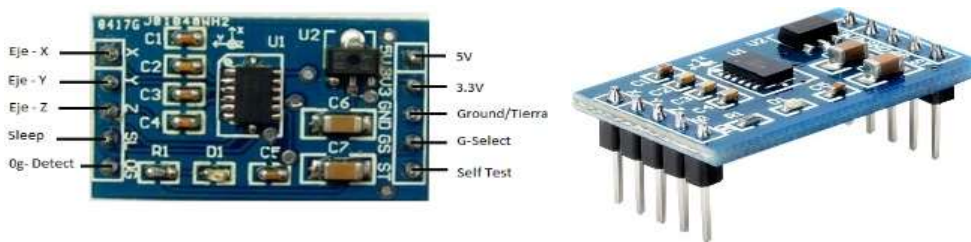
Acelerometro MMA7361 3 Ejes
