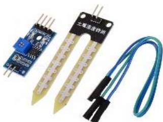
Humedad de Suelo YL-38
